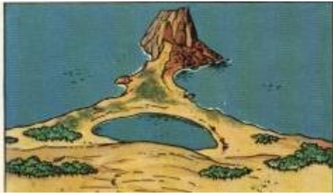
Peñón y tómbolo de Ifach
