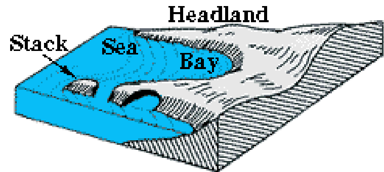
Aguja o pináculo costero (stack)
