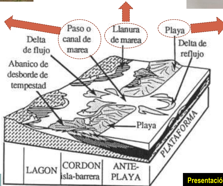
Llanura de marea
